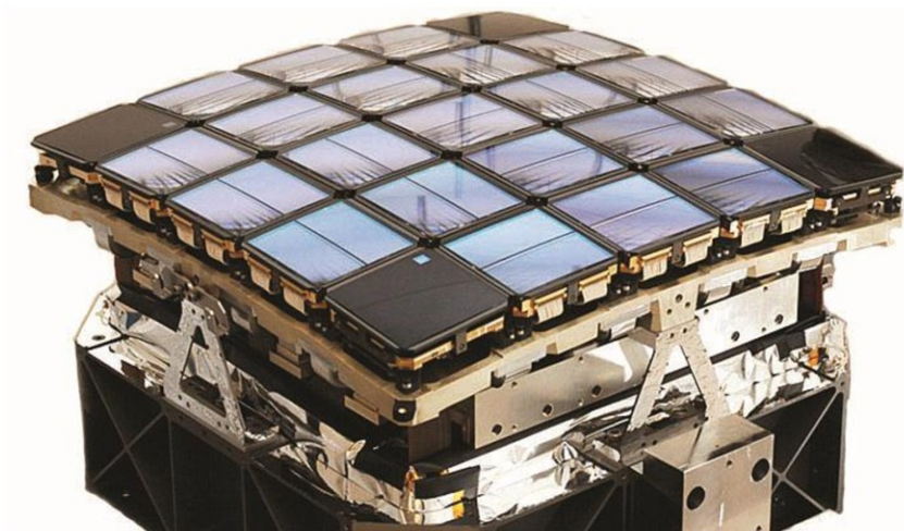
Matrice di 42 CCD di 2200 \times 1024 pixel ciascuno (95 Megapix)
